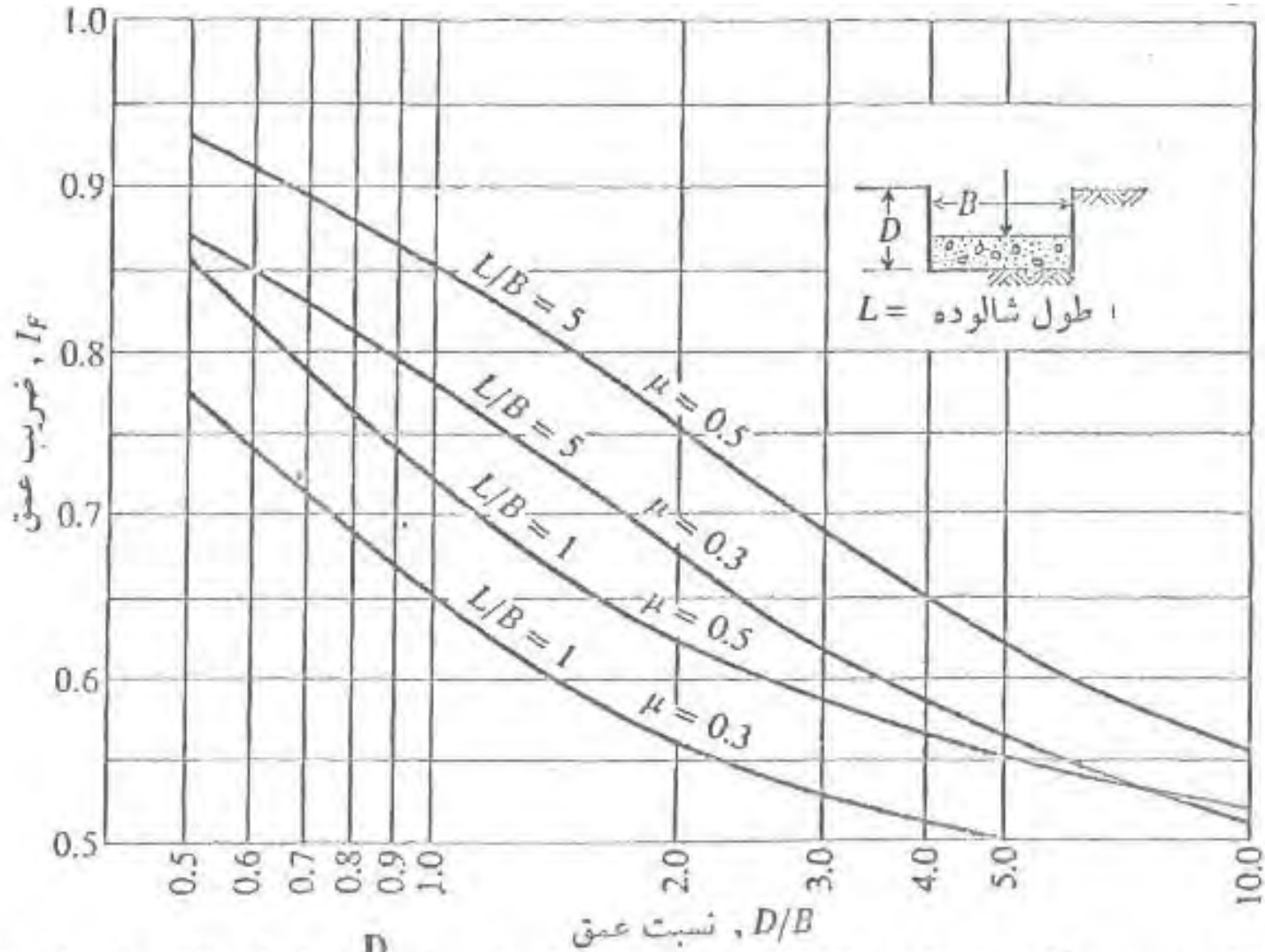
شکل (۵-۶). ضریب تأثیر I_F برای شالوده در عمق D . برای نسبت \frac{D}{B} از ابعاد واقعی استفاده نمائید
