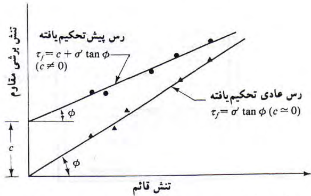
پوش گسیختگی خاک رس حاصل از آزمایش برش مستقیم زهکشی شده
