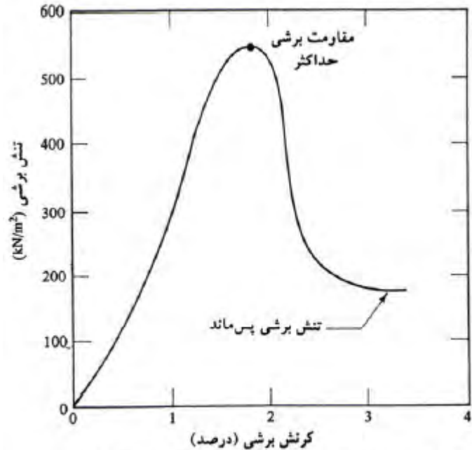
نتایج آزمایش برش مستقیم زهکشی شده بر روی رس پیش تحکیم یافته
