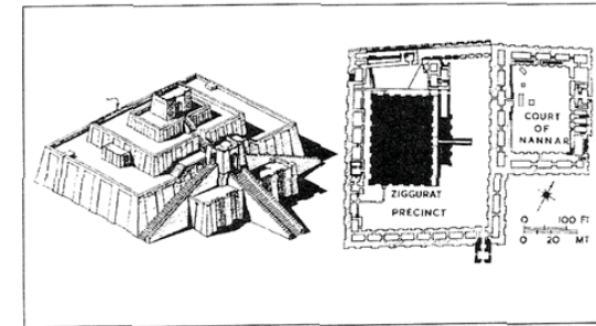
ش ۳- پرسکیو و پلان زیگورات اور (سومر)
